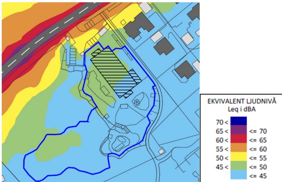
Ekvivalent ljudnivå. Observera att förskolegården med markerad blå linje har justerats (Efterklang 2022).
