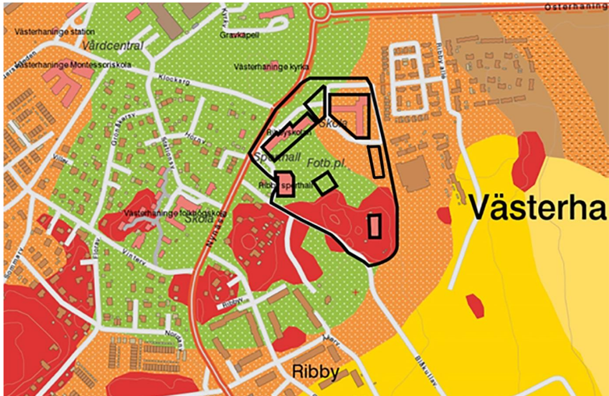
Föreslagna byggrätter svartmarkerade på den geotekniska kartan. Geoteknisk karta över planområdet, orange med vita prickar-postglacial finsand, grön med vita prickar-isälvsediment sand, röd-urberg, Sveriges Geotekniska Undersökning
