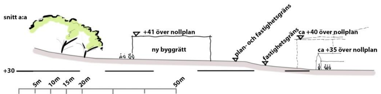
Snitt a:a illustrerar ny byggrätt i förhållande till Bovieran och angränsande radbus.
