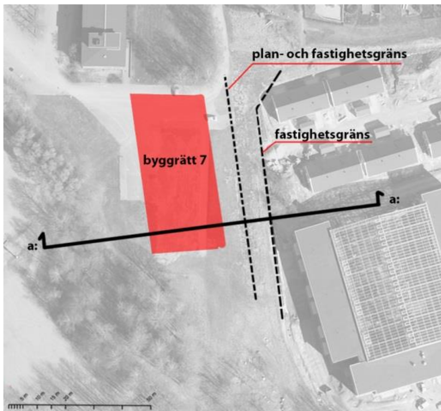
Läge för snitt a:a
