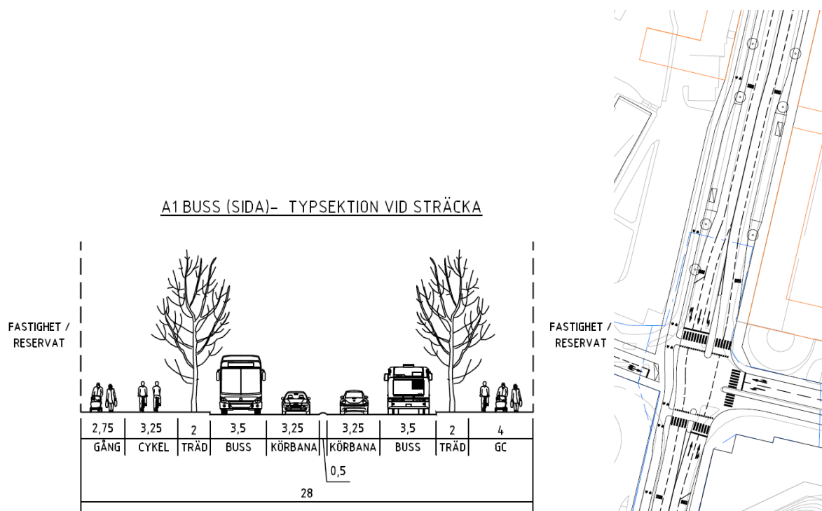
Figur 15. Gatusektion och planritning gata, i scenariot med separata busskörfält på Nynäsvägen. Korsningen som redovisas ovan är korsningen Nynäsvägen-Eskilsvägen. På gatsträckan finns också utpekade framtida hållplatsläge. Illustration: Sweco.
