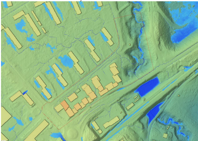
Figur 34. Framtida scenario, med föreslagen bebyggelse, vid ett skyfall med 66mm nederbörd och ingen infiltration. Planområdets ungefärliga läge är markerat med röd linje. Rinnstråk illustreras med blå linjer.
