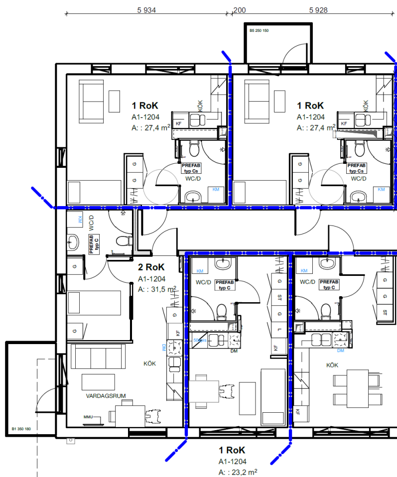
Figur 33. Möjlig planlösning med mindre lägenheter än 35 kvm för bebyggelsen närmast Åbyvägen
