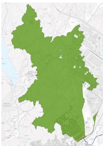
Figur 37. Planområdets (markerat i rött) läge inom det avrinningsområde som avvattnas mot Åbyån och den befintliga trumman, vid 75mm nederbörd.
