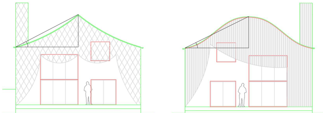
Figur 8 Illustration för vägledning av beräkning för takvinkel för principiella sadeltak med konkavt respektive sinuskurveformat takfall.
