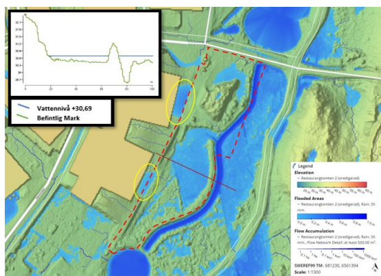
Figur 10. Marköversvämning vid dämningnivå +30,69 möh motsvarande 35 mm regn, som motsvarar säkerhetsnivå 3.
