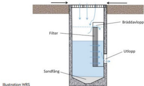
Figur 25. Principskiss brunnsfilter.
