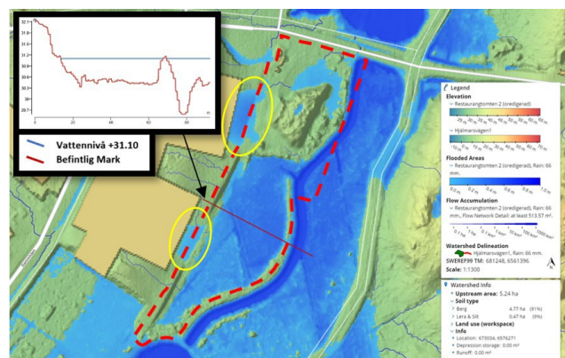
Figur 11. Marköversvämning vid dämningnivå +31,10 möh motsvarande säkerhetsnivå 3.
