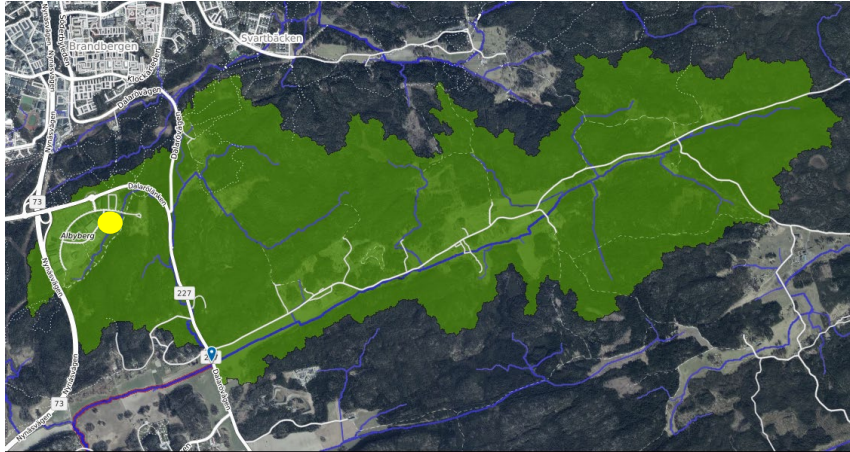
Figur 21. Avrinningsområdet som avrinner mot fastigheterna Alby 2:3, Hässlingby 21:1, Alby 1:9-4, Hässlingby 18:3-1. Detaljplaneområdet visas med gul markering.
