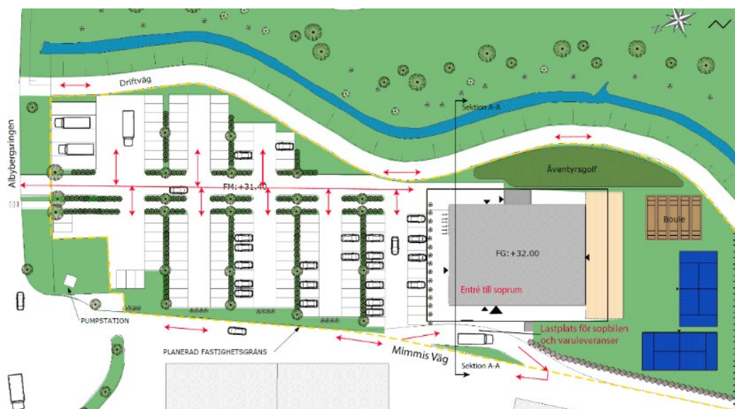
Figur 16. Illustrationsbild med möjliga trafikrörelser och hur angöring sker till bebyggelsen samt för sopbil och varuleveranser med sektion A-A för figur 17.
