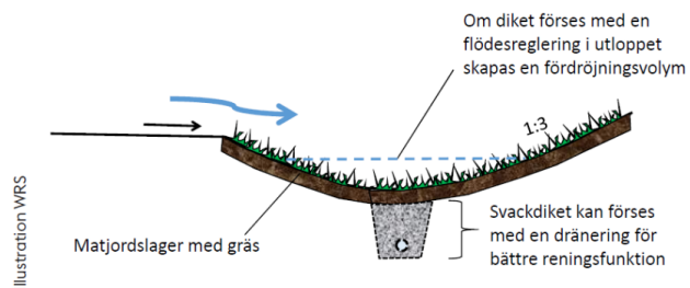
Figur 26. En principskiss för ett svackdike. Svackdiken etableras i nivå under ytan som ska avvattas
