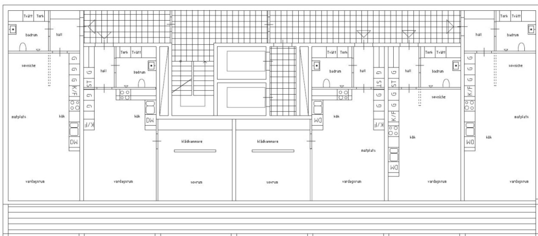
Bild 42: Exempel på planlösningar för byggnaderna ovanför centrumbyggnaden.
