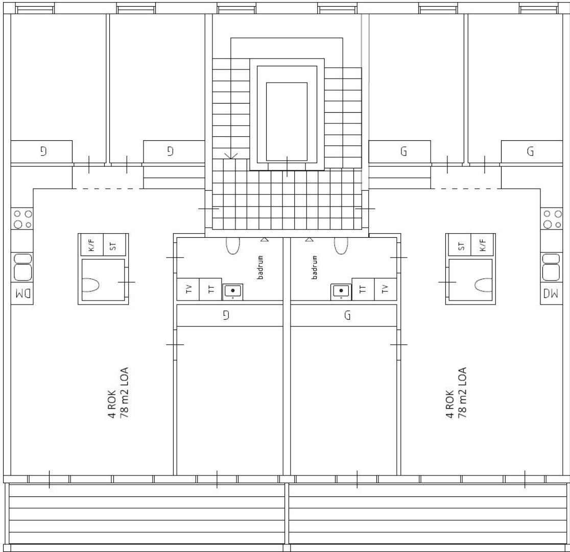
Bild 41: Exempel på planlösning för huset mot Norra Kronans gata. White Arkitekter AB
