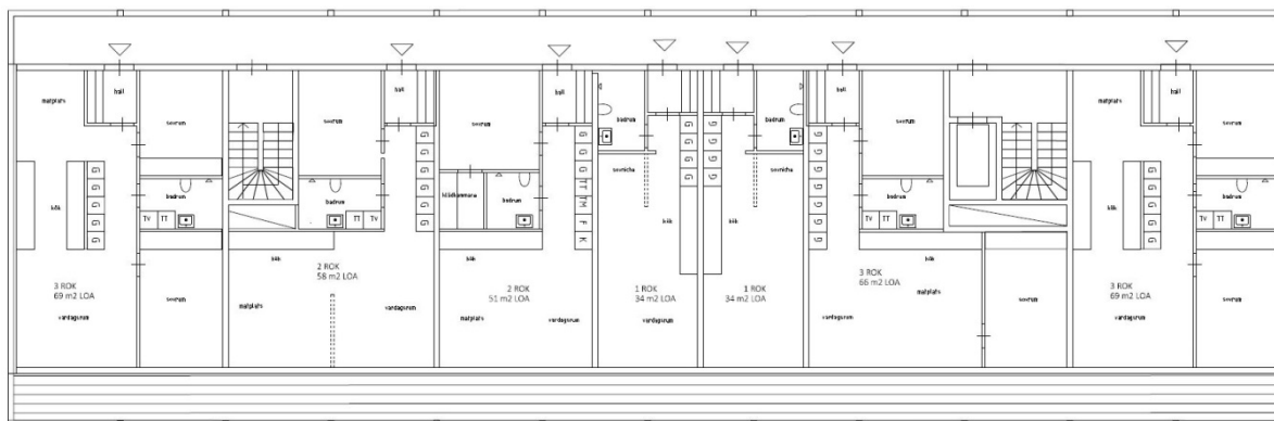
Bild 40: Exempel på planlösningar för husen med fasad mot Brandbergsleden. Loftgången är vänd mot gata, uteplatser är vända mot innergården och tyst sida. White Arkitekter AB
