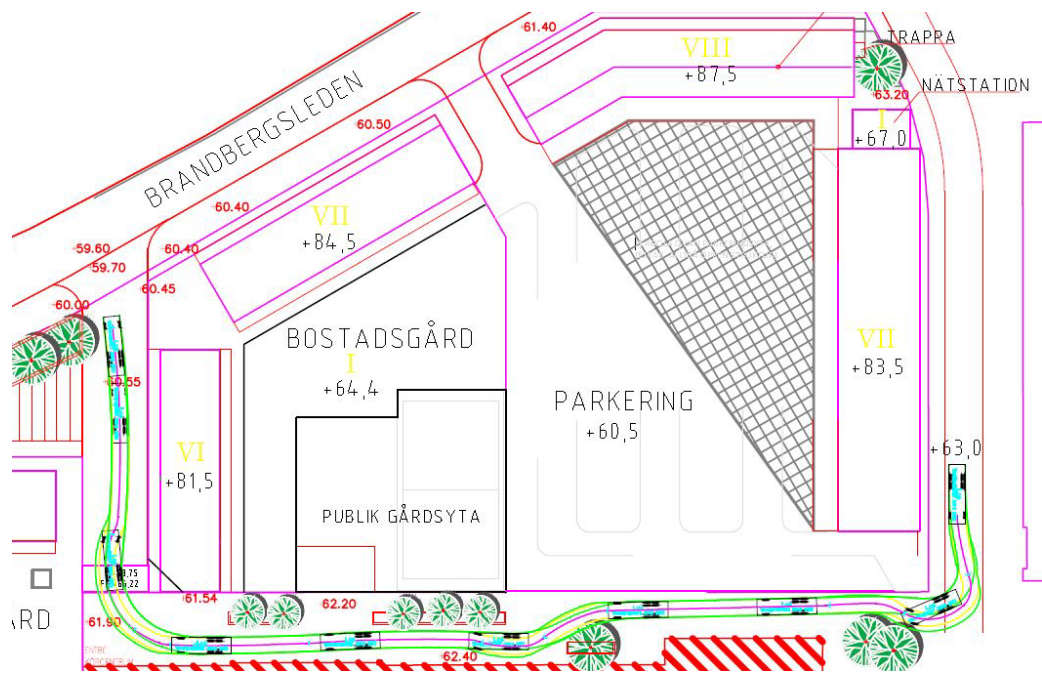
Bild 44: Utdrag ur projekteringsunderlaget som visar hur ett körfält för sopbilar kan se ut. Illustration White Arkitekter AB.
