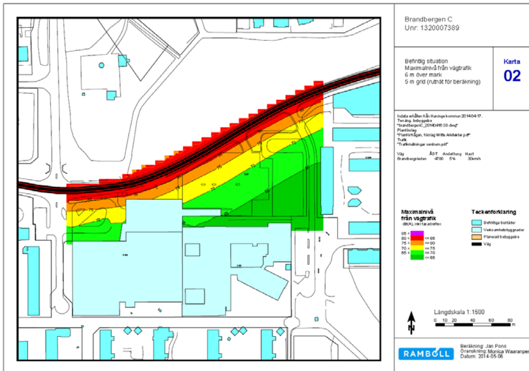
Bild 12: Bullerkarta maximalnivå från vägtrafik.
