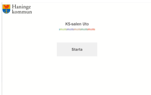
Figur 1 Startsida
