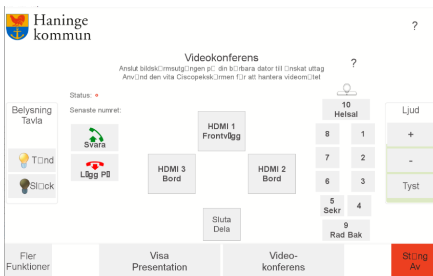
Figur 5 Vy Videomöte
