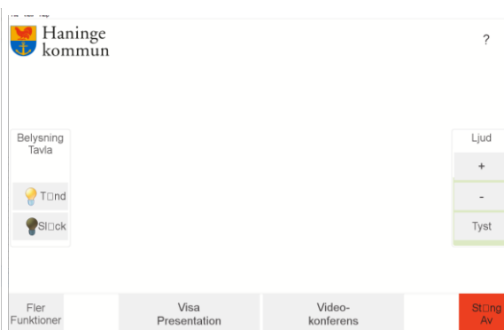
Figur 2 Huvudsida
